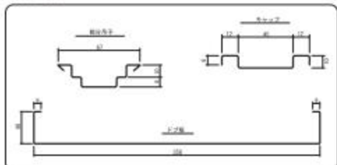
断面形状図
