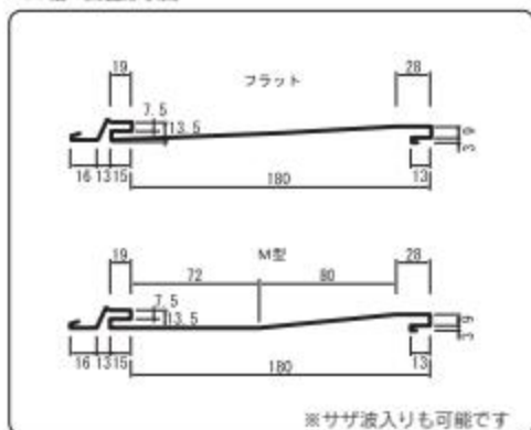
180幅 断面形状図
