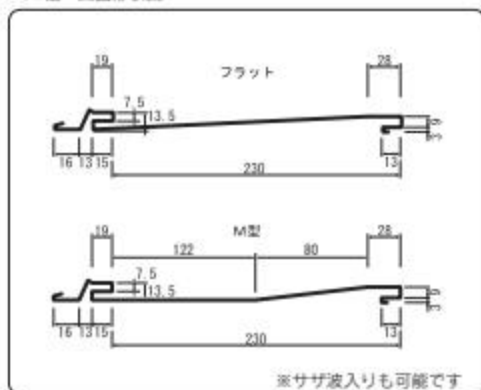
230幅 断面形状図
