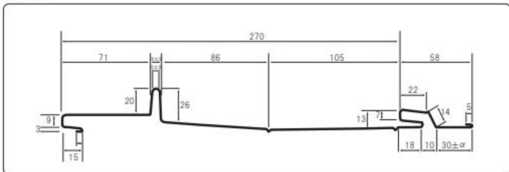
断面形状図
