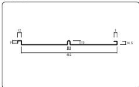
断面形状図
