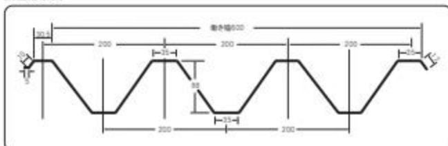
断面形状図
