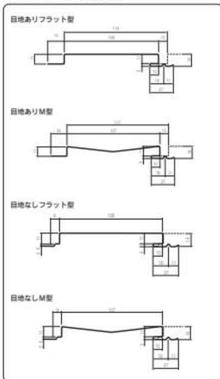
スパンドレル I型 断面形状図
